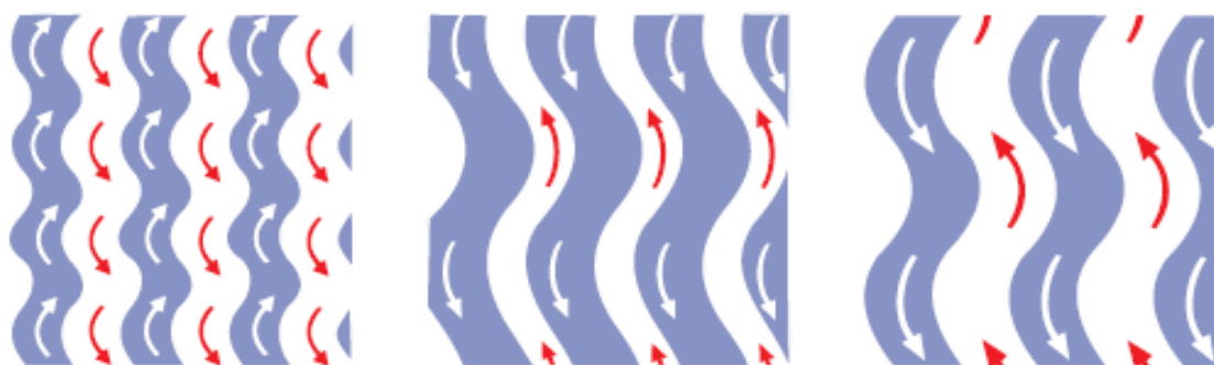
Примеры схем потоков в теплообменниках Free Flow
