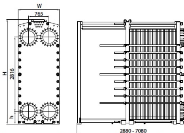
Габаритный чертеж, Размеры в мм
