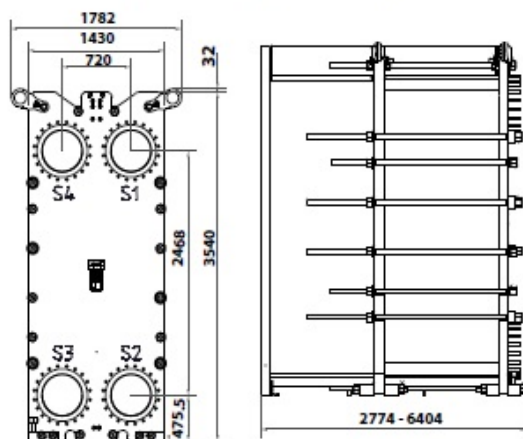
Габаритный чертеж, Размеры в мм
