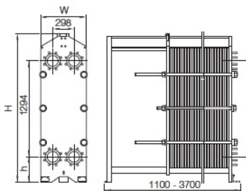
Габаритный чертеж, Размеры в мм
